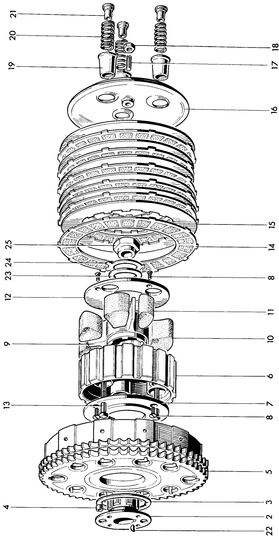
Fig. 10. CLUTCH
