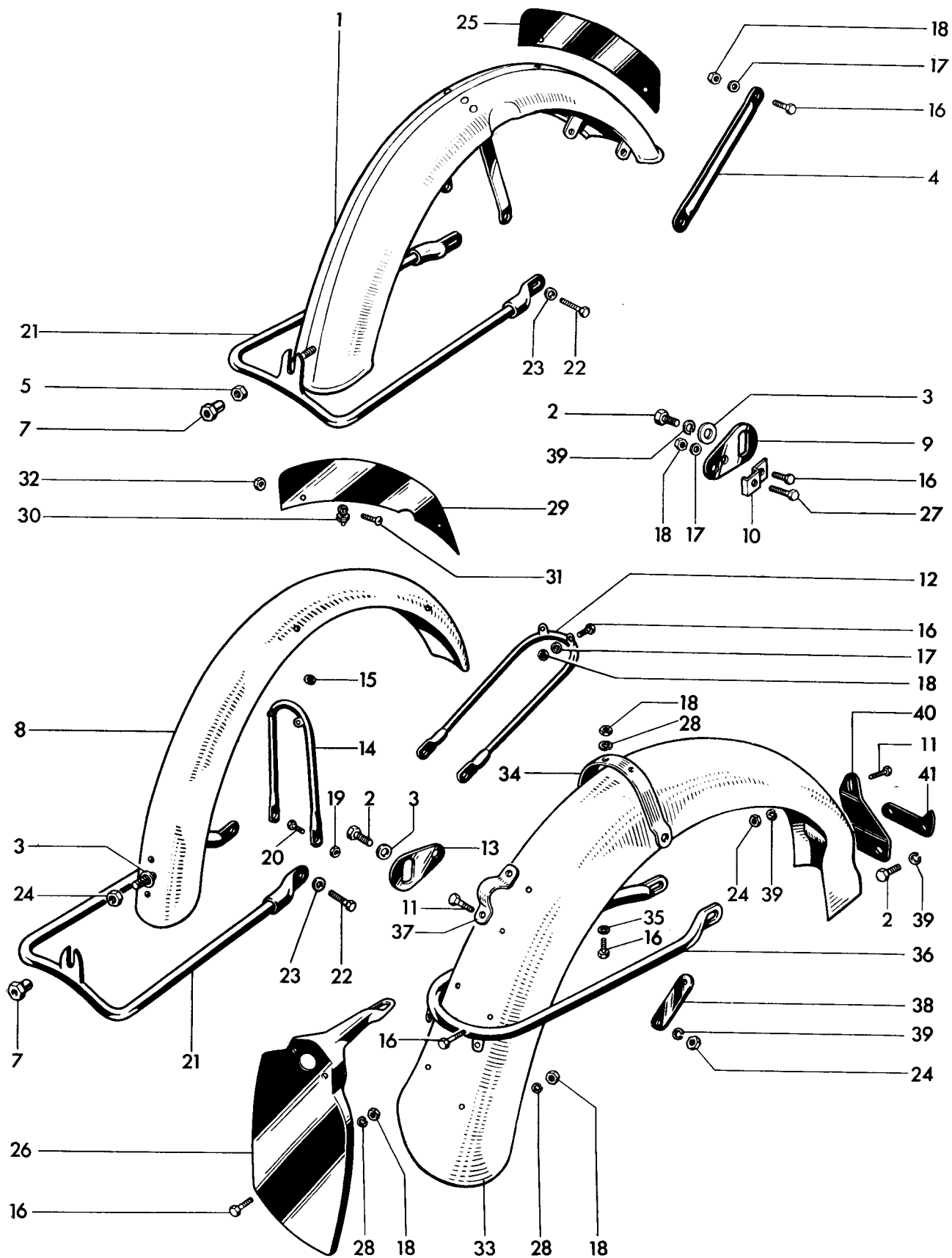
Fig. 26. MUDGUARDS
